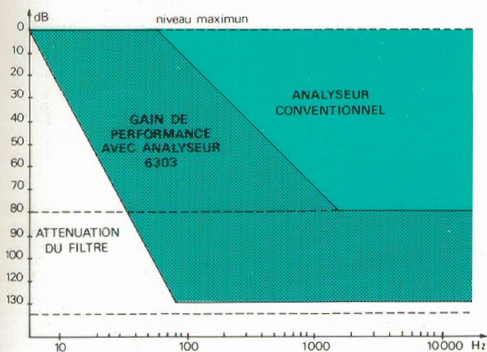
Cette figure illustre le gain de performance en dynamique et en résolution de l'analyseur ADRET (courbe noire) par rapport aux analyseurs classiques (courbe couleur), dans le cas de l'analyse d'un même signal.
