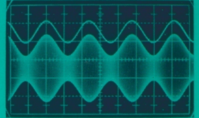
Modulation d'amplitude
