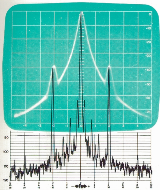
Cette figure illustre le gain de performance en dynamique et en résolution de l'analyseur ADRET (courbe noire) par rapport aux analyseurs classiques (courbe couleur), dans le cas de l'analyse d'un même signal.
