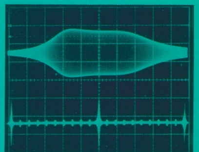
Modulation d'un filtre large bande centré sur 1,04 MHz. (Marqueurs tous les 10 kHz).
