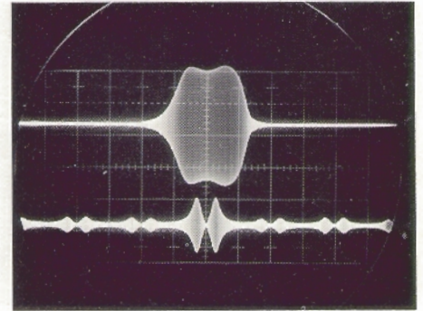
Fig. 3 - WOBULATION D'UN FILTRE A QUARTZ 250 kHz
